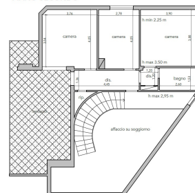
PIANO SECONDO
