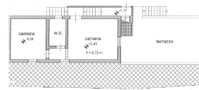
PIANTA PIANO TERRA
