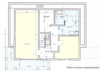
Piano terreno-seminterrato
